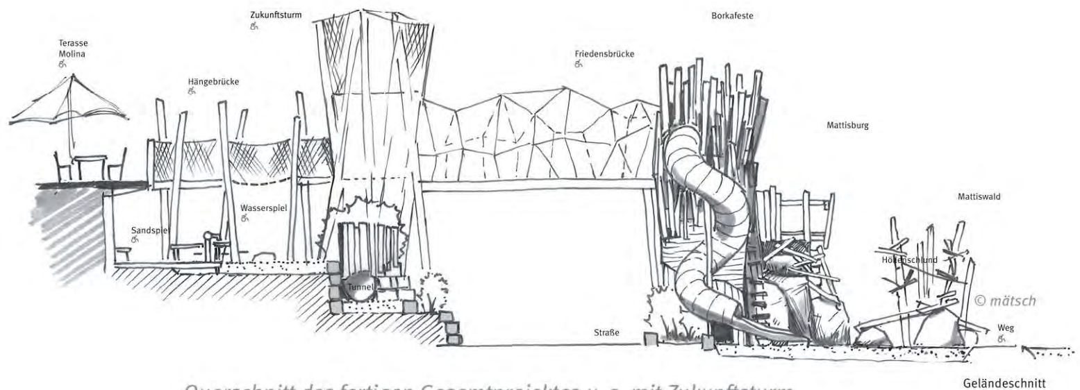
Querschnitt des fertigen Gesamtprojektes u. a. mit Zukunftsturm, Friedensbrücke und Mattisburg mit Kellergang und Röhrenrutsche u.v.m.
